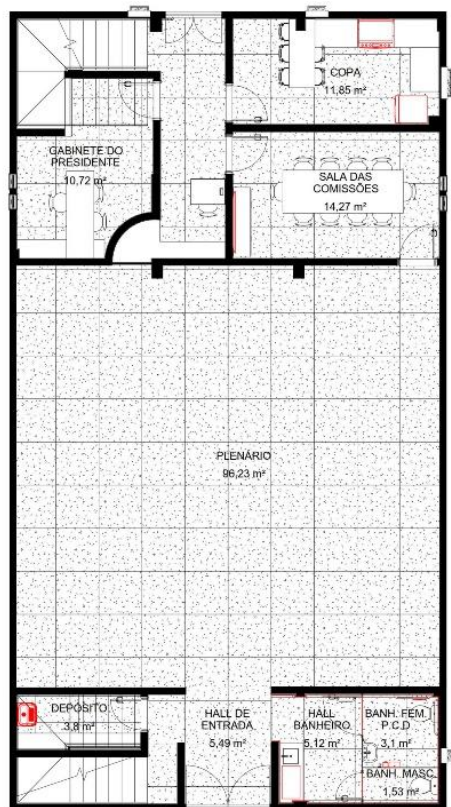
PLANTA DE LAYOUT 1º PAVIMENTO ESCALA: 1/100
