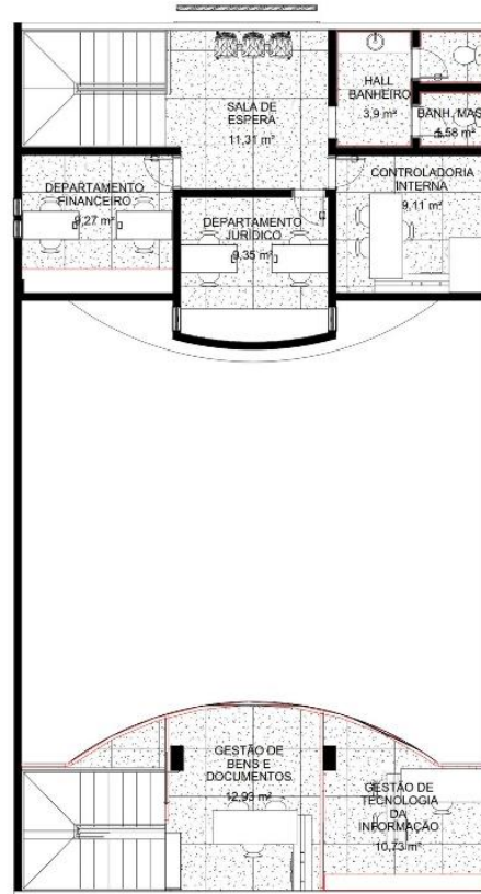
PLANTA DE LAYOUT 2º PAVIMENTO ESCALA: 1/100
